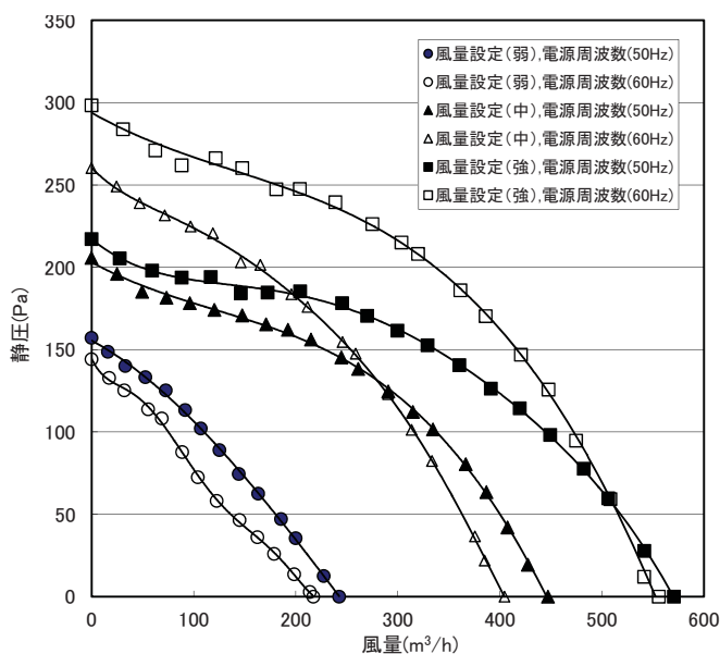
風量 - 静圧曲線
