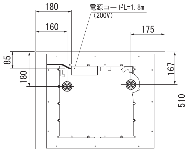
背面図
