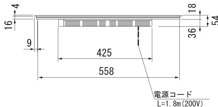
正面図
