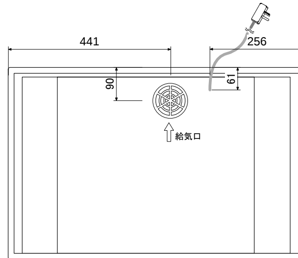
底 面 図
