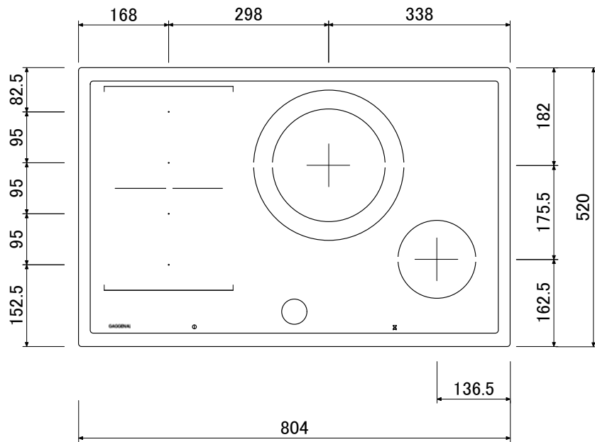
上 面 図
