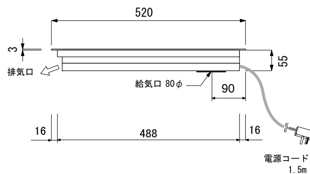
側 面 図
